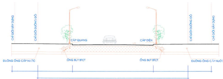
MẶT CẮT 2-2
