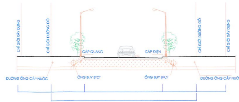
MẶT CẮT 3-3
