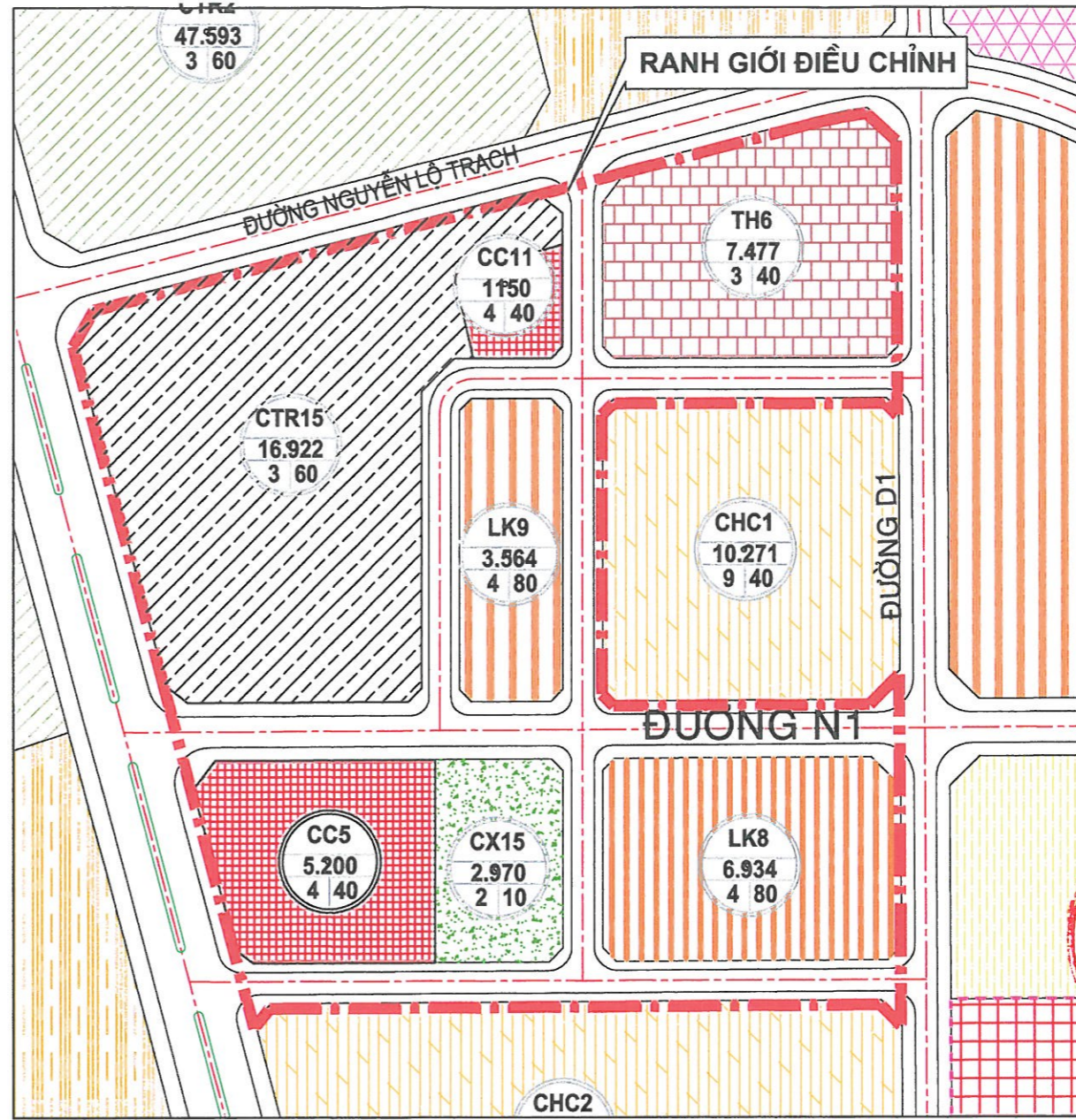
BẢN VẼ ĐIỀU CHỈNH QUY HOẠCH
