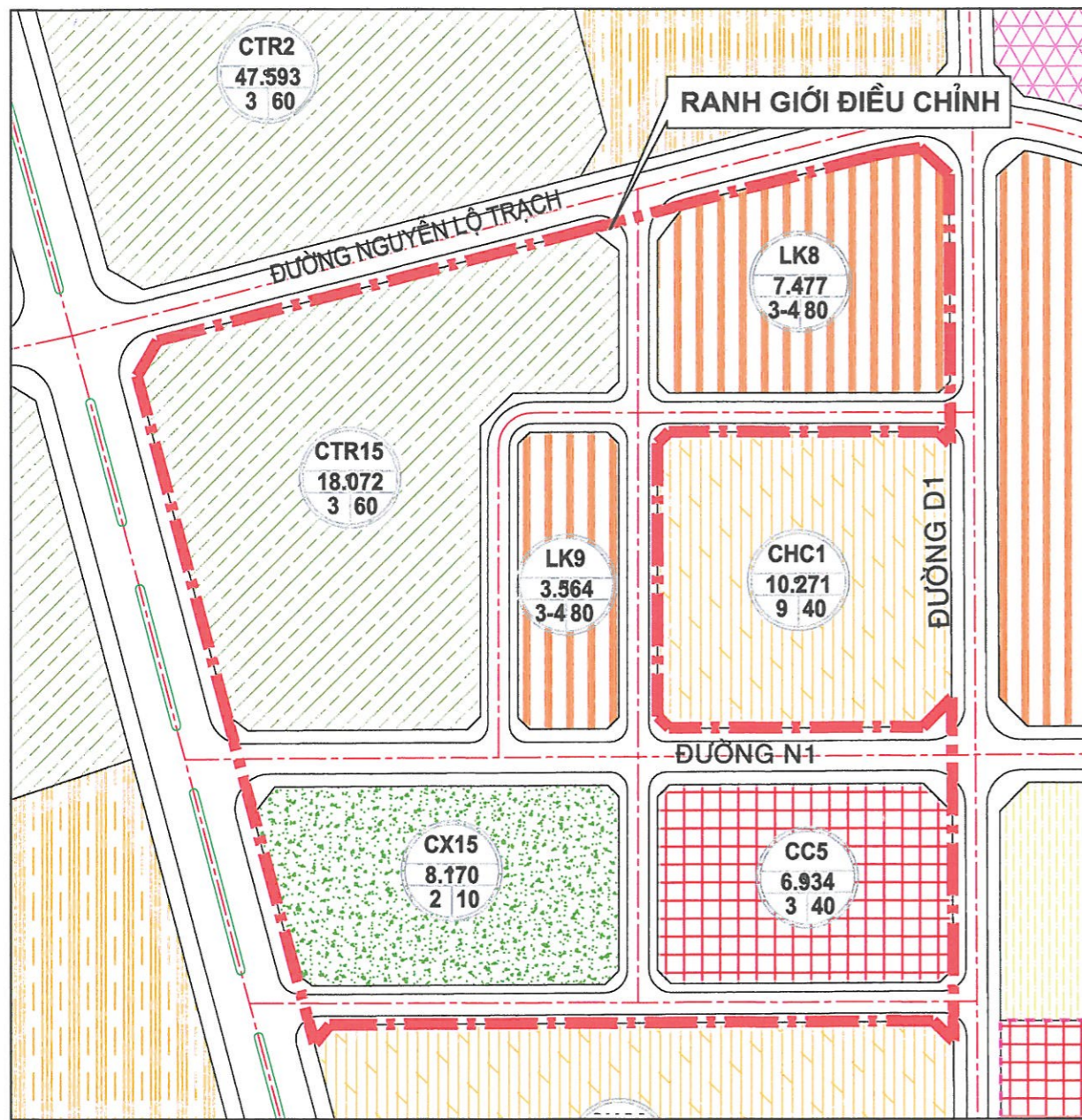
BẢN VẼ QUY HOẠCH (ĐÃ PHÊ DUYỆT)
