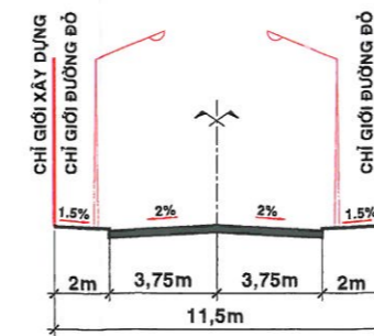
MẶT CẮT 1-1: TỶ LỆ 1/200
