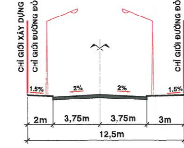
MẶT CẮT 2-2: TỶ LỆ 1/200
